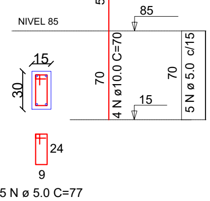
PILARES 15X30
