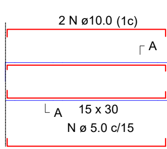
VIGAS (15X30)
