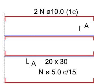
VIGAS (20X30)
