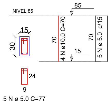
PILARES 15X30 MORRE
