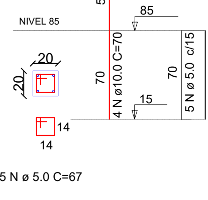
PILARES 20X20
