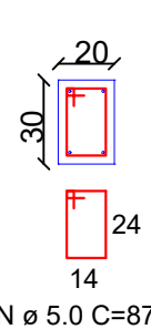
SEÇÃO A-A
