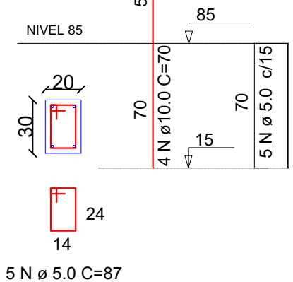
PILARES 20X30
